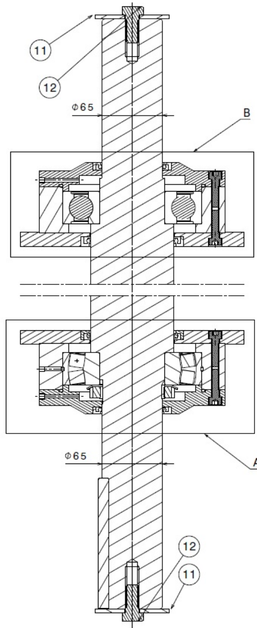
Front view Scale: 1:4
